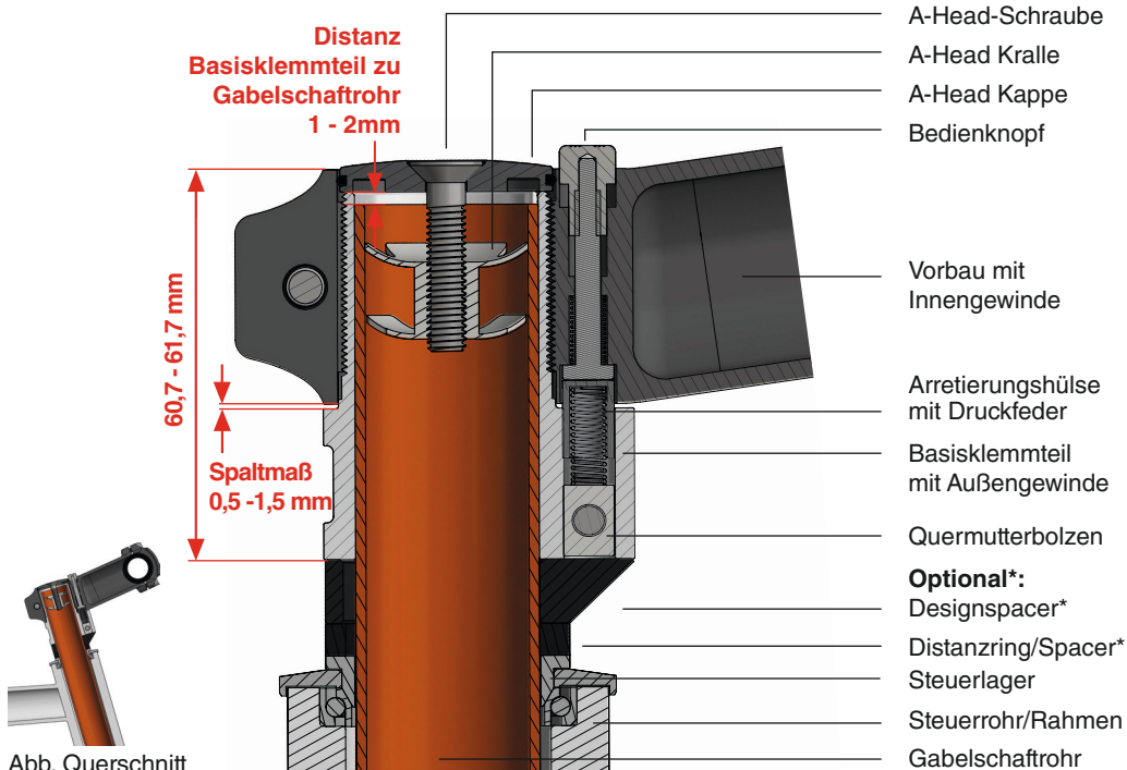
Abb. Querschnitt
